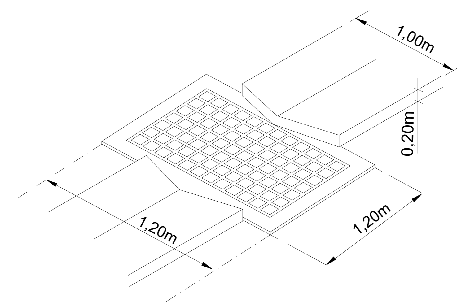
Detalhes da caixa com grade
