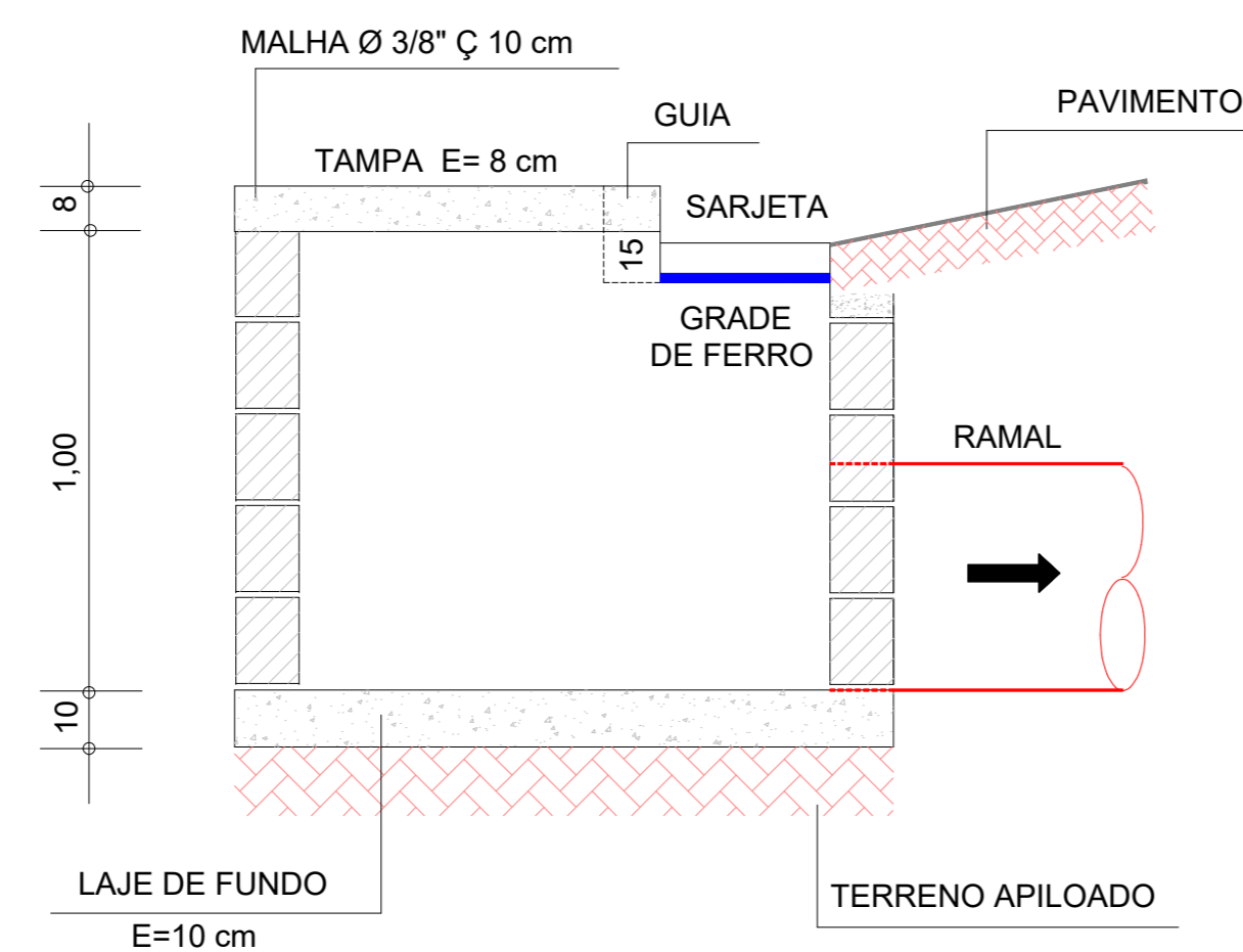
CORTE B-B ESCALA: 1:20
