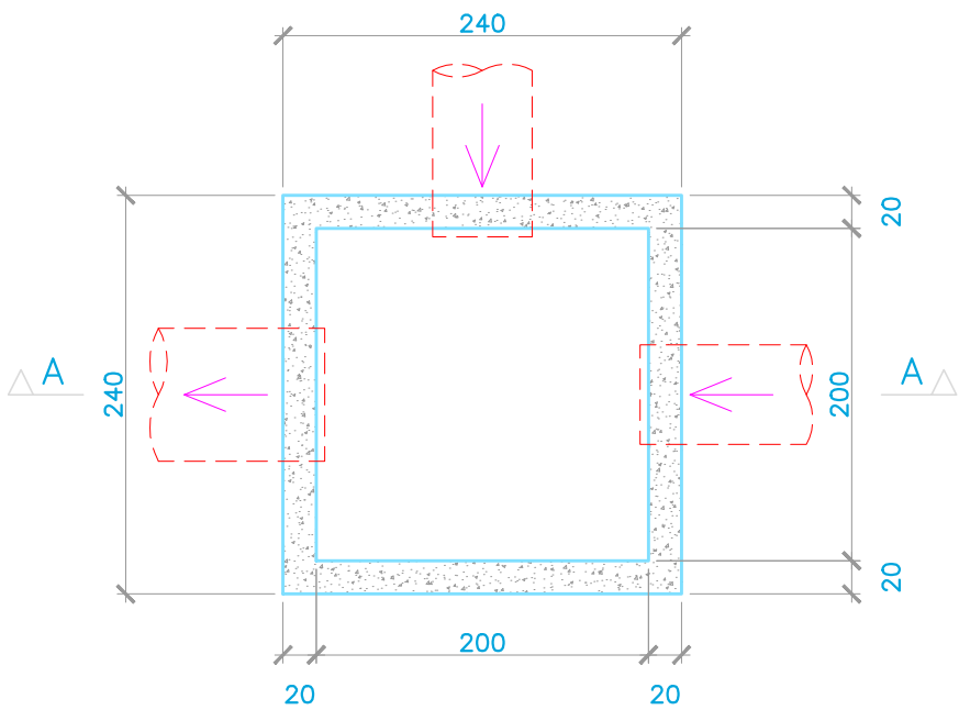
FÔRMA VISTA SUPERIOR Esc: 1/50
