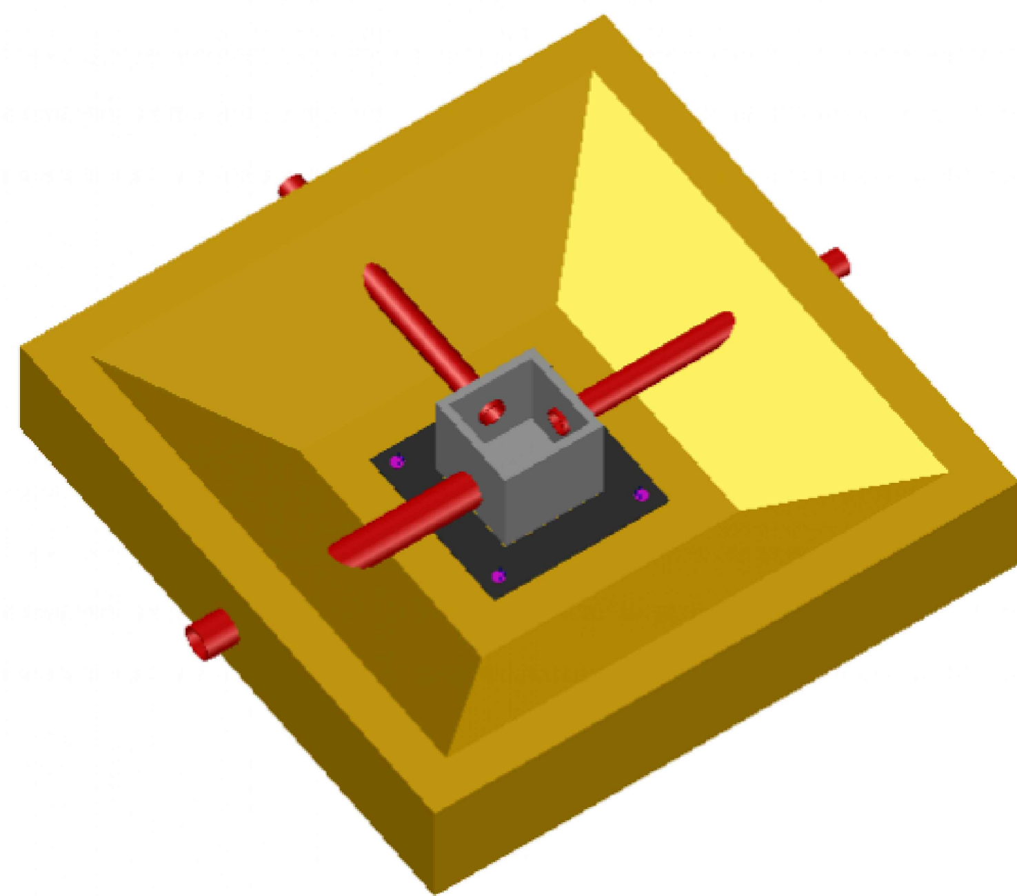
2- EXECUÇÃO DAS ESTACAS E CONCRETO MAGRO.
