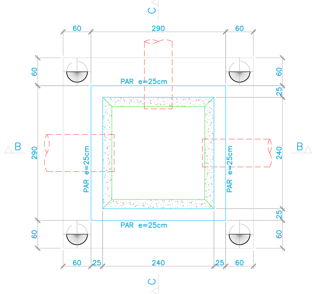
FÔRMA VISTA SUPERIOR Esc: 1/50
