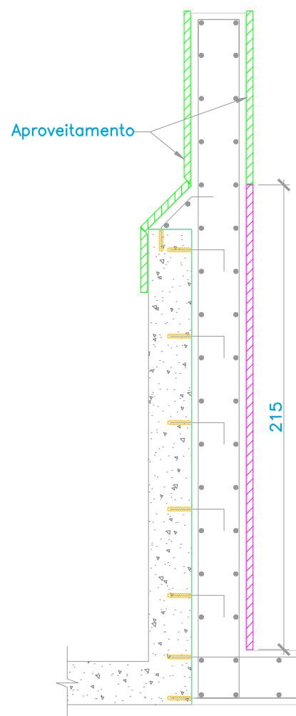
DETALHE TÍPICO EXECUÇÃO DE FÔRMA Esc: 1/25
