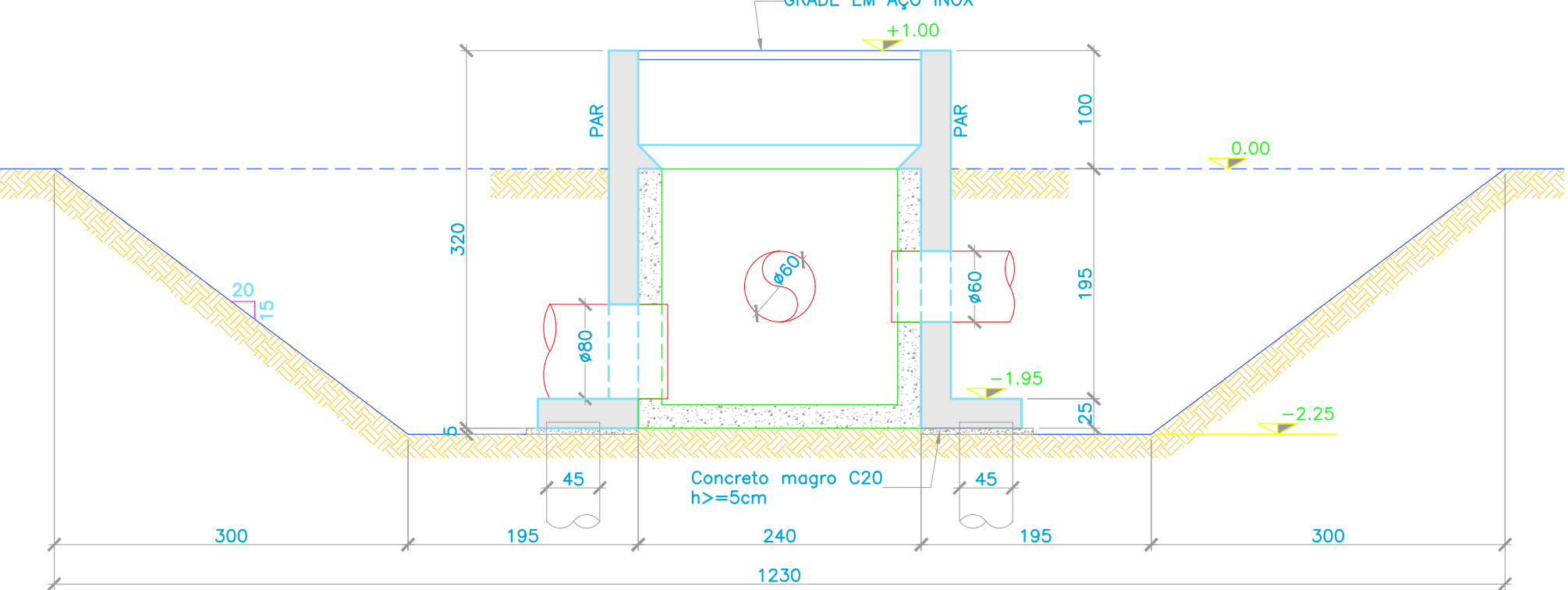
Corte B-B
