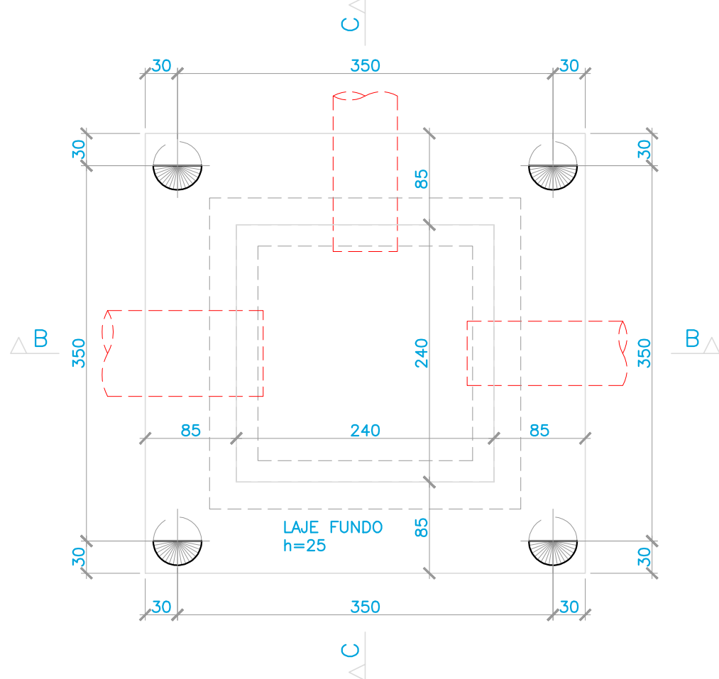
LOCAÇÃO DAS ESTACAS Esc: 1/50
