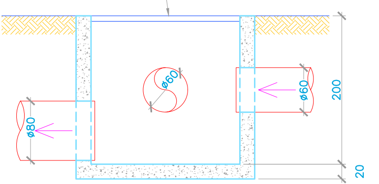
Corte A-A
