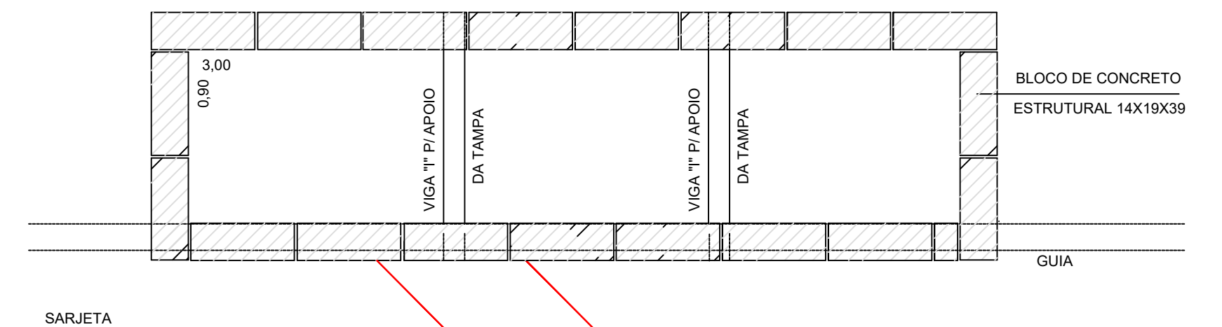
REBAIXO DA SARJETA
