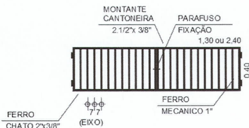
Figura 2: Grade de ferro com sistema basculante padrão SAECIL
