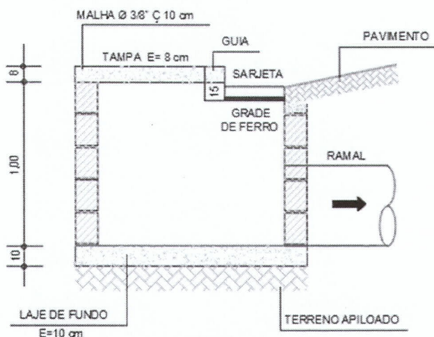
Figura 1: Boca de lobo padrão SAECIL
