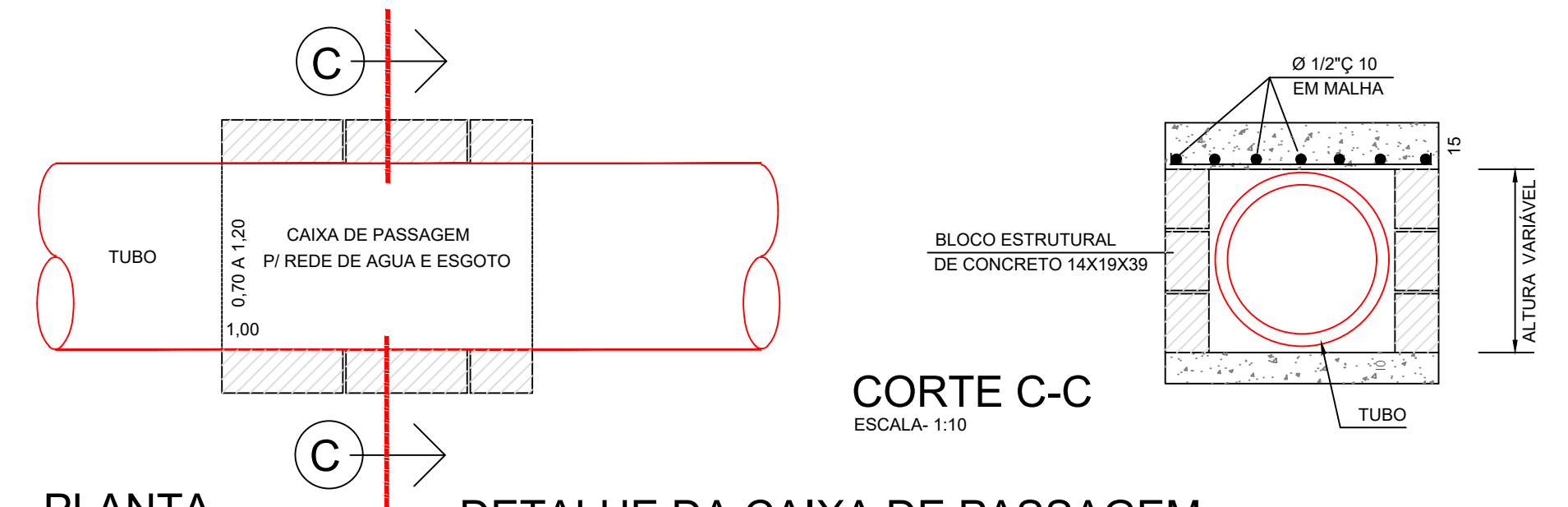
DETALHE DA CAIXA DE PASSAGEM
